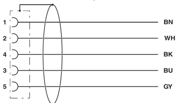
Kontaktbelegung des M12-Buchse
