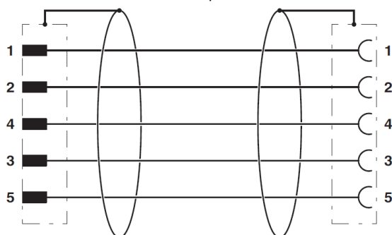
Kontaktbelegung des M12-Stecker und der M12-Buchse
