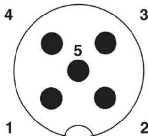
Polbild M12-Stecker, 5-polig, A-kodiert, Ansicht Stiftseite
