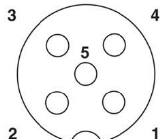
Polbild M12-Buchse, 5-polig, A-kodiert, Ansicht Buchsenseite
