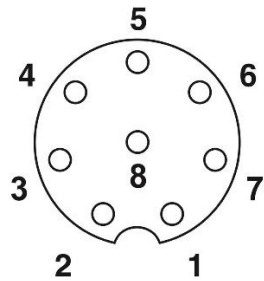
Polbild M12-Buchse, 8-polig, A-kodiert, Ansicht Buchsen­seite
