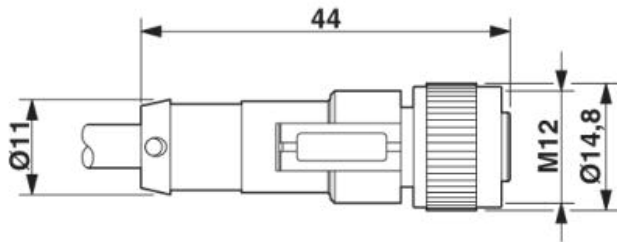
Buchse M12 x 1, gerade
