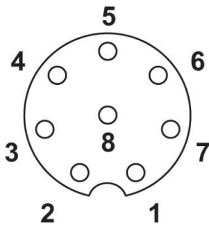
Polbild M12-Buchse, 8-polig, Ansicht Buchsenseite
