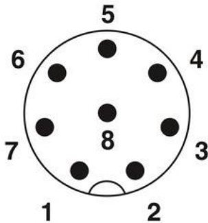
Polbild M12-Stecker, 8-polig, A-kodiert, Ansicht Stiftseite
