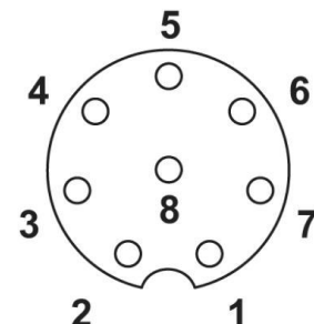
Polbild M12-Buchse, 8-polig, A-kodiert, Ansicht Buchsen­seite
