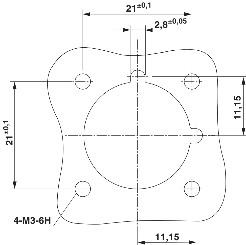
Bohrplan/Lötpadgeometrie
