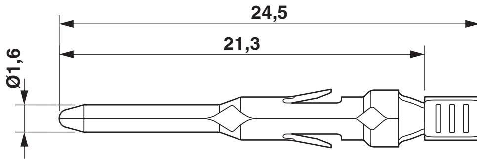
Maßzeichnung
