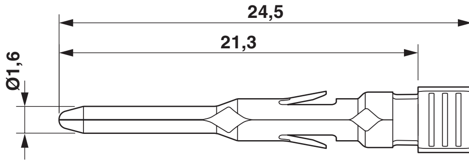
Maßzeichnung
