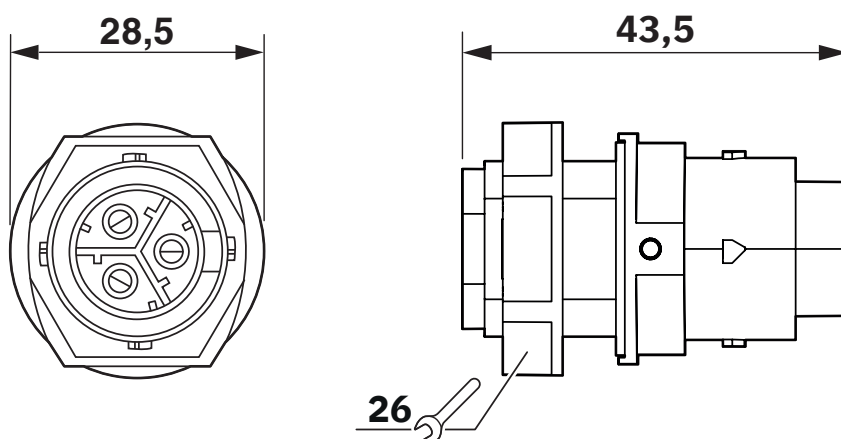
Maßzeichnung
