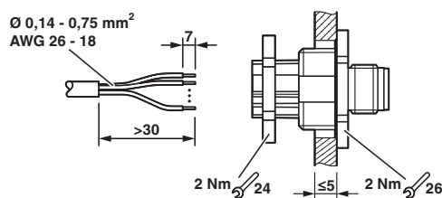
Funktionszeichnung
