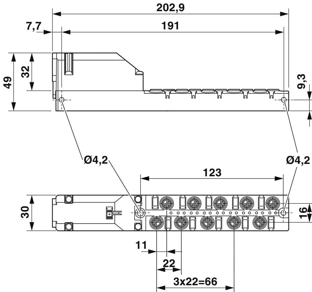
Maßzeichnung
