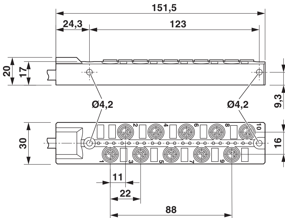
Maßzeichnung
