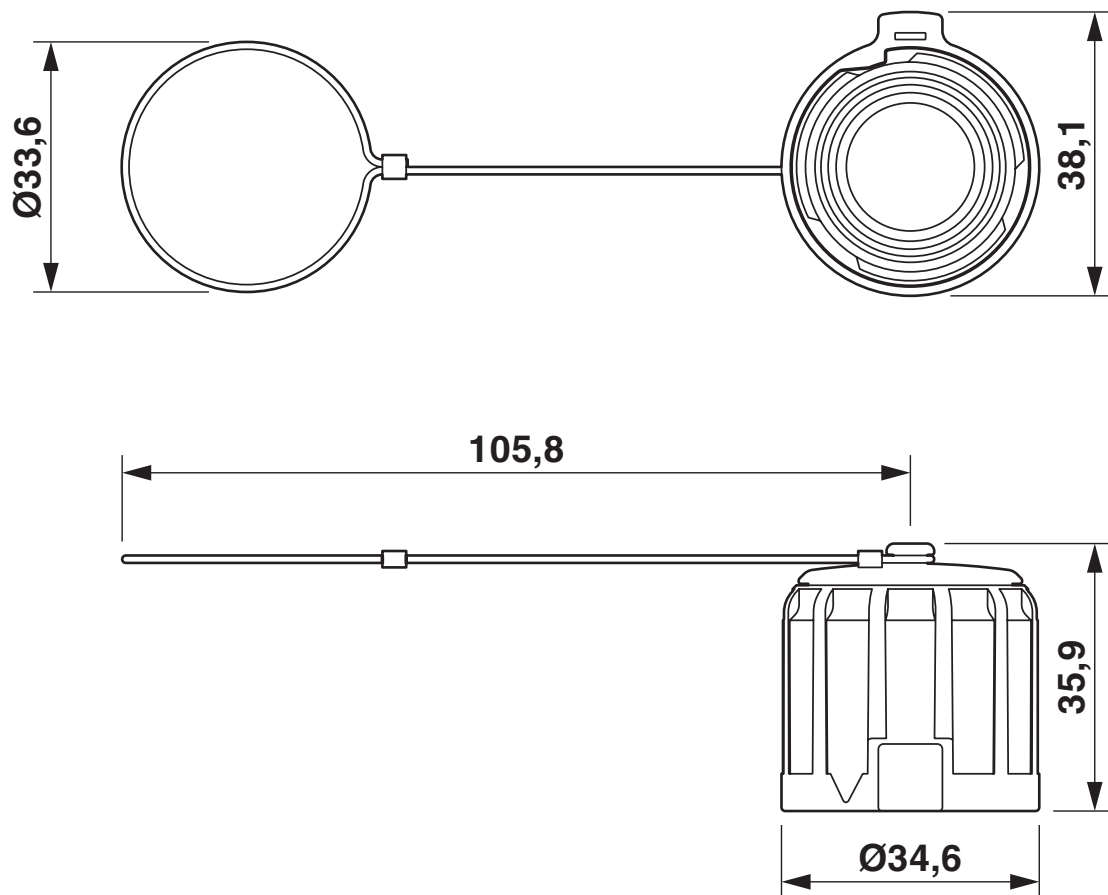
Maßzeichnung
