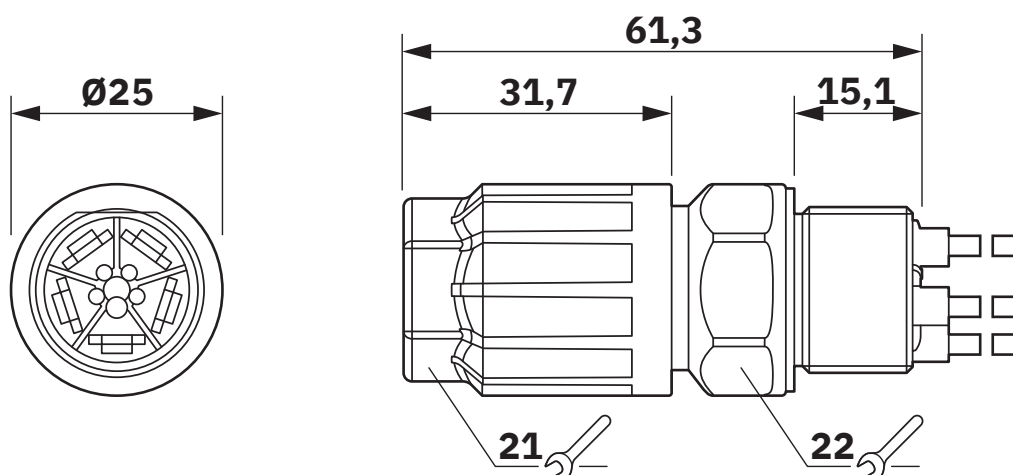
Maßzeichnung
