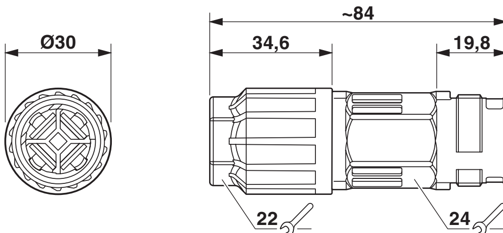
Maßzeichnung
