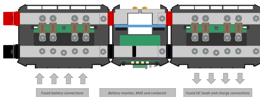
Lynx Smart BMS mit zwei Lynx-Verteilern
