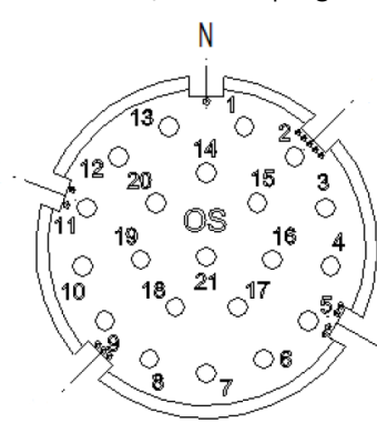
00008747 E-Part / Stift 21 polig
