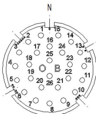
00008978 P-Part / Buchse 26 polig
