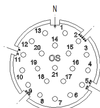
00009082 E-Part / Stift 21 polig
