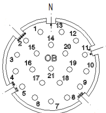
00009135 P-Part / Buchse 21 polig
