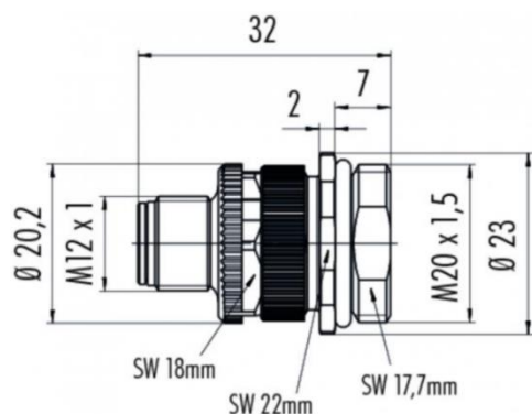
Flanschstecker
