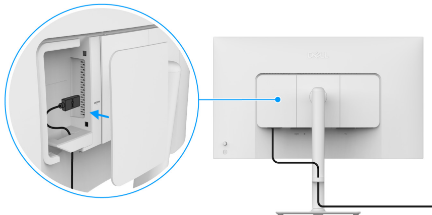
Abbildung 22. Anbringen der seitlichen E/A-Abdeckung
