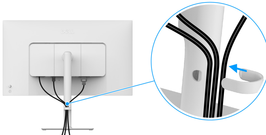
Abbildung 23. Kabel verlegen
