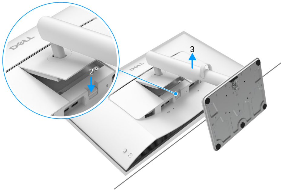
Abbildung 26. Entfernen des Monitorständers
