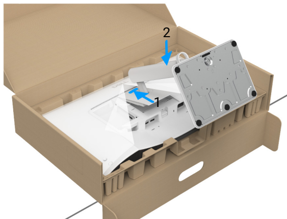
Abbildung 16. Befestigung des Ständers am Monitor
