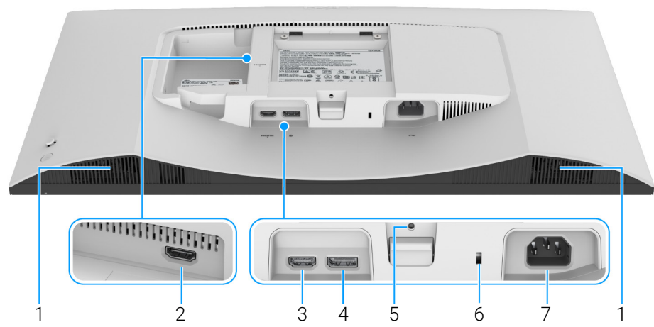
Abbildung 4. Ansicht von unten ohne Monitor-Standfuß
