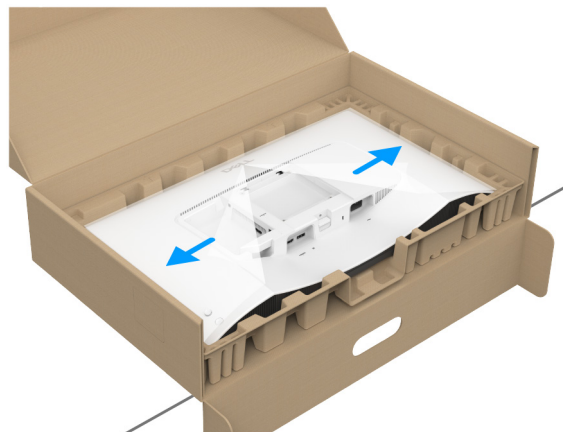
Abbildung 15. Öffnen der Schutzabdeckung
