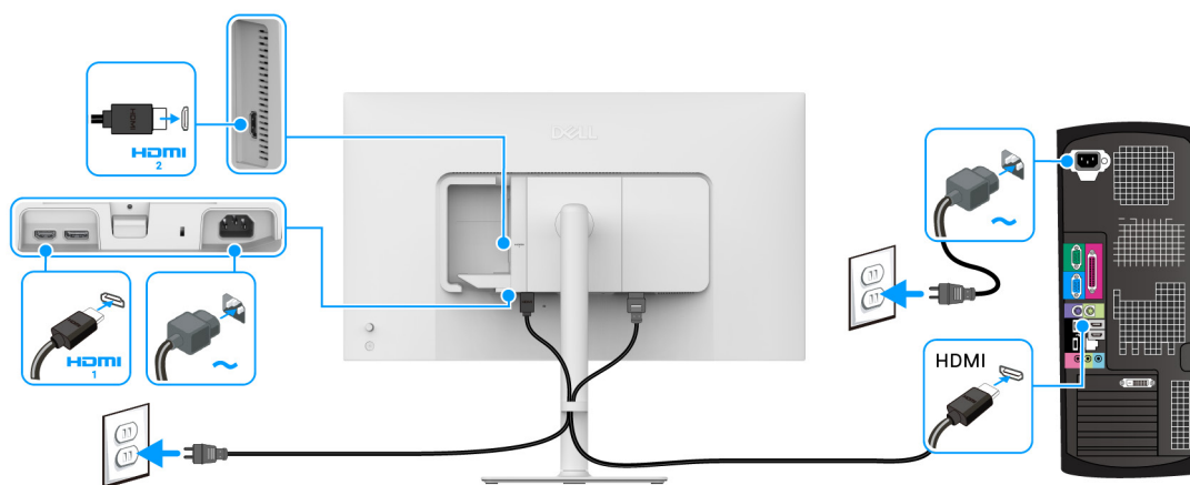
Abbildung 19. HDMI Verbindung
