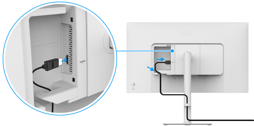
Abbildung 21. Verlegen der Kabel
