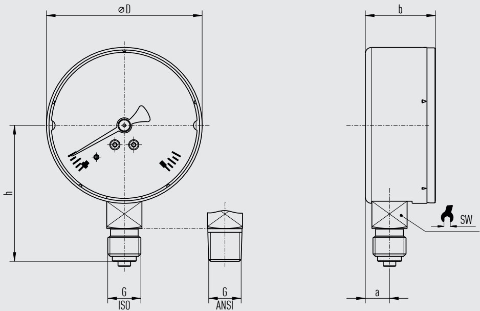
Typ 131.11, Anschluss radial unten
