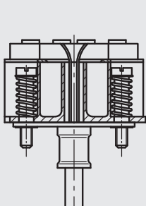
Messeinsatz mit aufgebautem Transmitter (hier: Typ T32)
