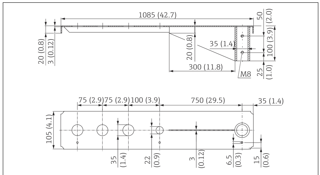
33 Abmessungen Ausleger 1 000 mm schwenkbar für Sensor Prozessanschluss Kabeleinführung. Maß- heit mm (in)
