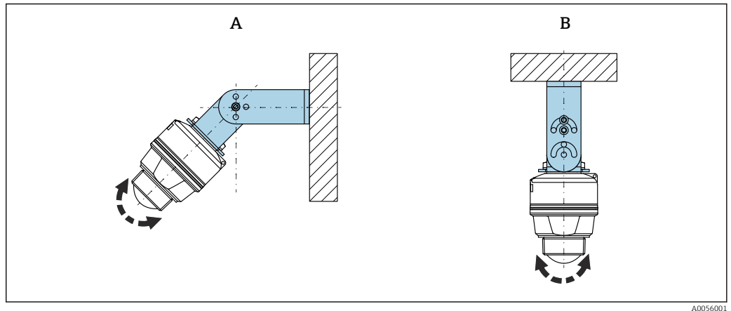
6 Einbau mit Montagebügel ausrichtbar
