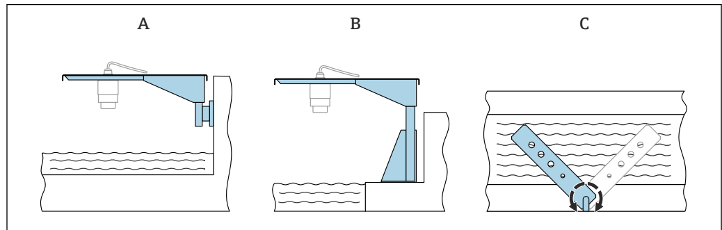
8 Montage Ausleger schwenkbar
