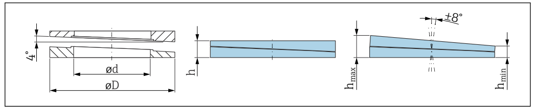
45 Abmessungen
