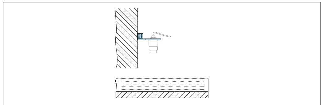
9 Ausleger mit Wandhalter, schwenk- und verschiebbar (z. B. um das Gerät auf die Mitte einer Messrinne auszurichten)
