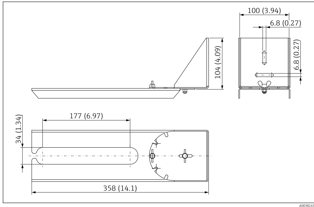
40 Abmessungen schwenkbare Montagehalterung. Maßeinheit mm (in)
