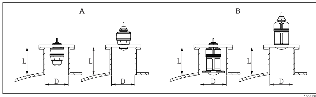
3 Stutzenmontage
