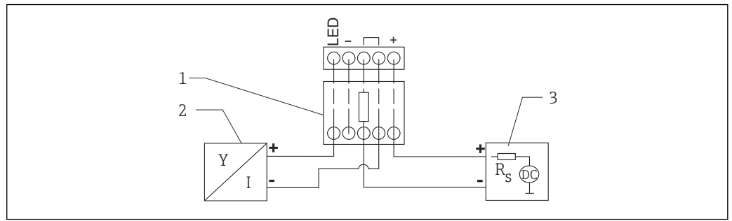
15 Blockschaltbild HART-Gerät, RIA15 mit Beleuchtung, HART-Kommunikationswiderstandsmodul
