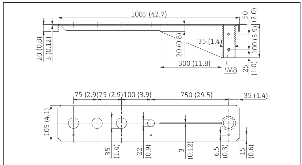
41 Abmessungen Ausleger 1 000 mm schwenkbar für Sensor Prozessanschluss Kabeleinführung. Maßeinheit mm (in)
