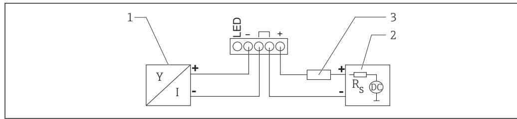
12 Blockschaltbild HART-Gerät mit Prozessanzeiger RIA15 ohne Beleuchtung
