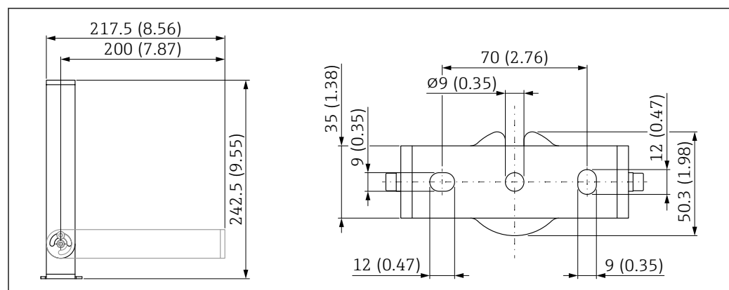
36 Abmessungen Montagebügel. Maßeinheit mm (in)
