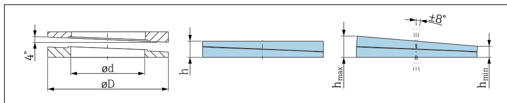
56 Abmessungen
