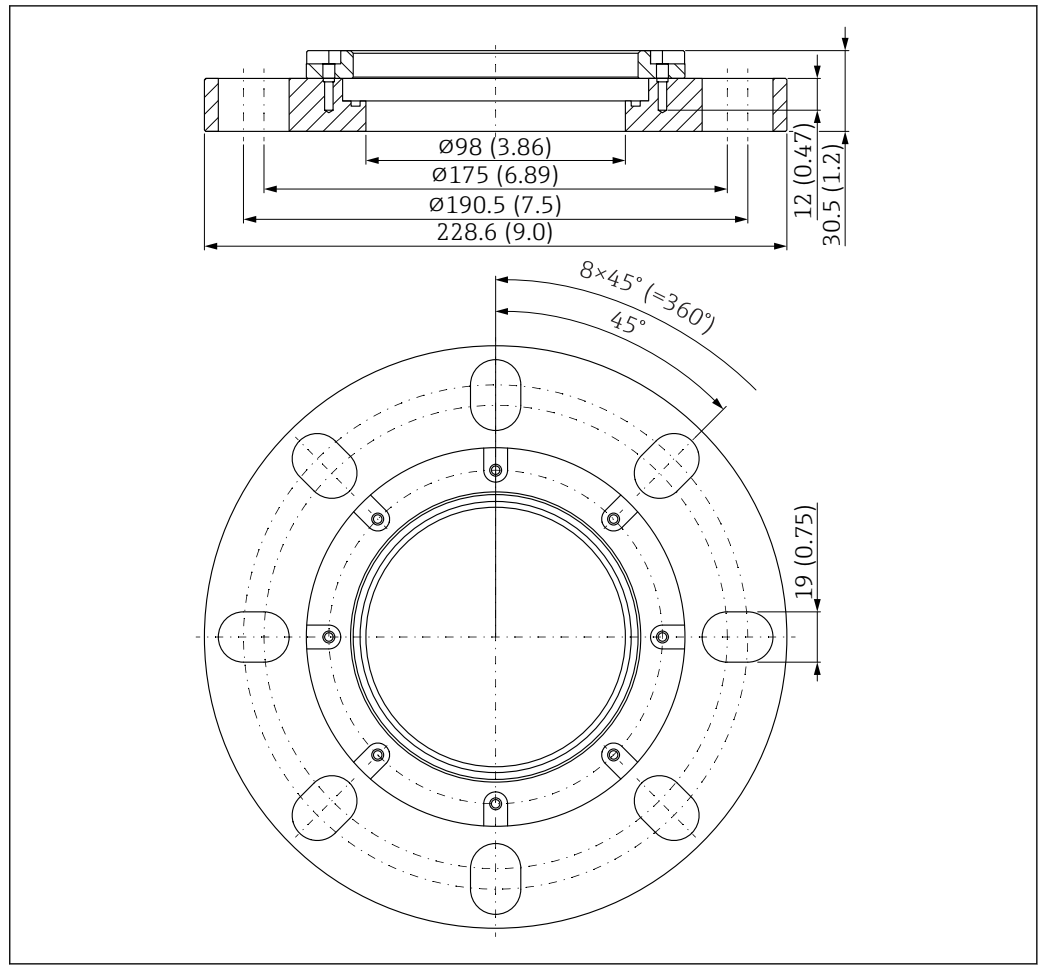
51 Abmessungen UNI-Überwurfflansch 4"/DN100/100. Maßeinheit mm (in)
