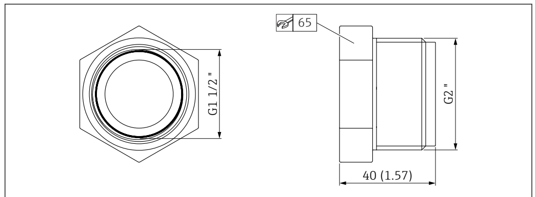
30 Abmessungen Adapter Uni
