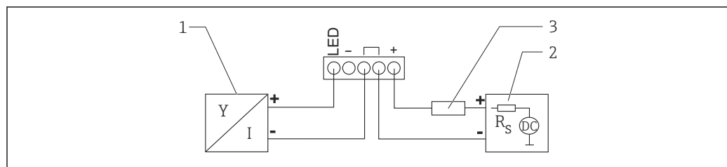
13 Blockschaltbild HART-Gerät mit Prozessanzeiger RIA15 mit Beleuchtung
