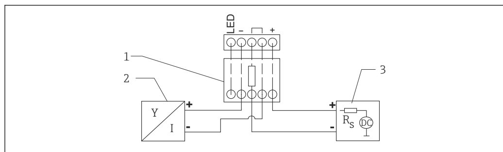
14 Blockschaltbild HART-Gerät, RIA15 ohne Beleuchtung, HART-Kommunikationswiderstandsmodul
