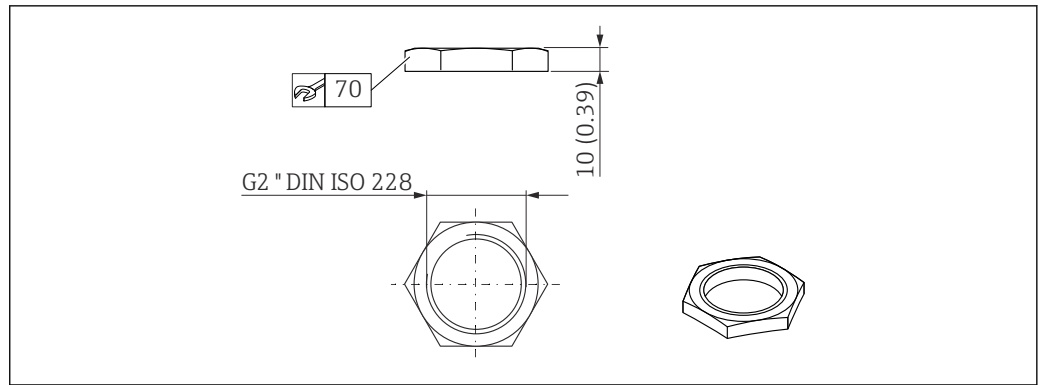
29 Abmessungen Befestigungsmutter. Maßeinheit mm (in)
