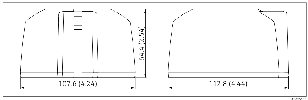
26 Abmessungen für Wetterschutzhaube G1/NPT1, Kabeleinführung von oben. Maßeinheit mm (in)
