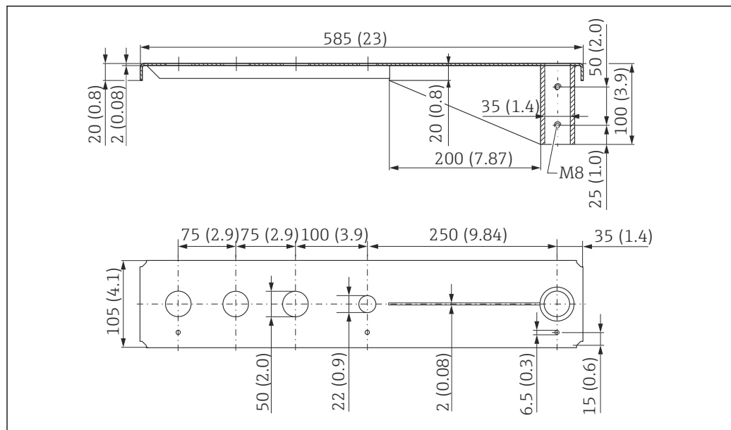
43 Abmessungen Ausleger 500 mm schwenkbar für Sensor Prozessanschluss Antennenende G 1½". Maßeinheit mm (in)
