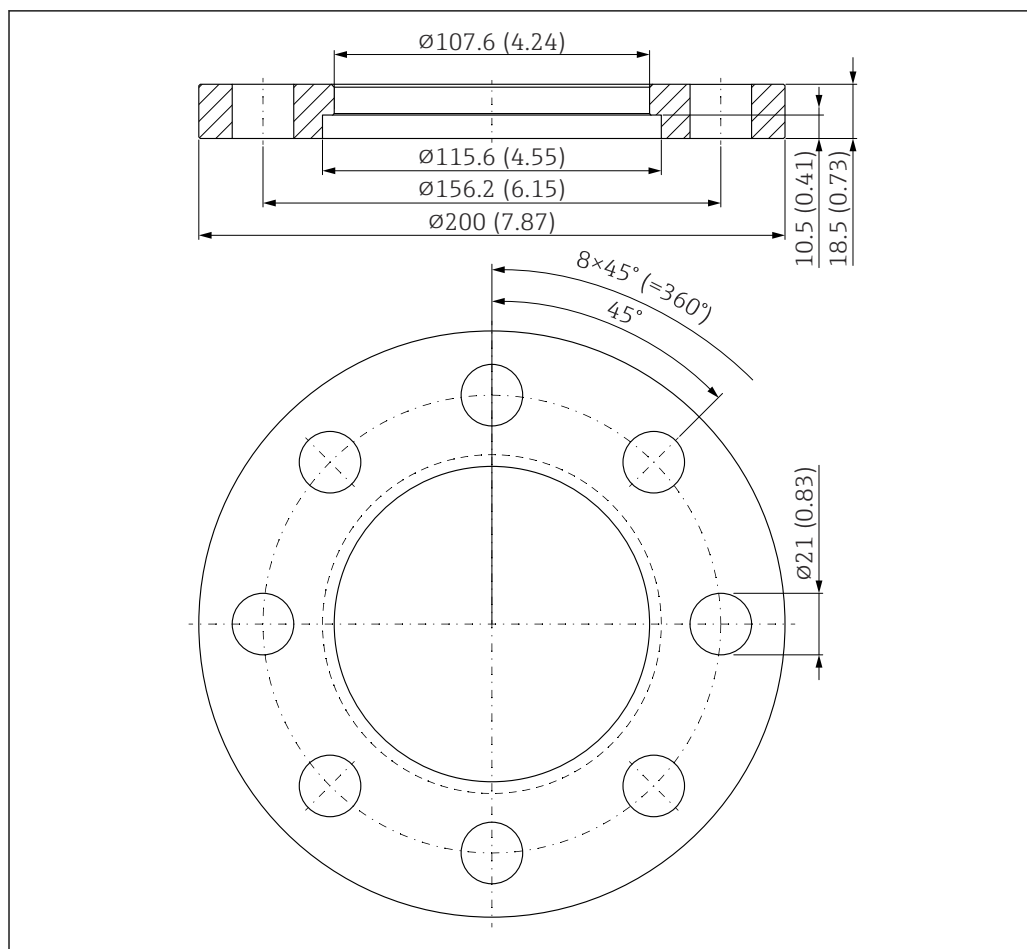
50 Abmessungen UNI-Überwurfflansch 3"/DN80/80. Maßeinheit mm (in)
