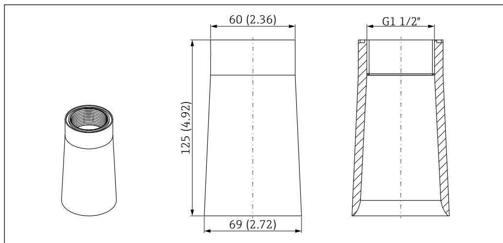
32 Abmessungen Überflutungsschutzhülse 40 mm (1,5 in). Maßeinheit mm (in)
