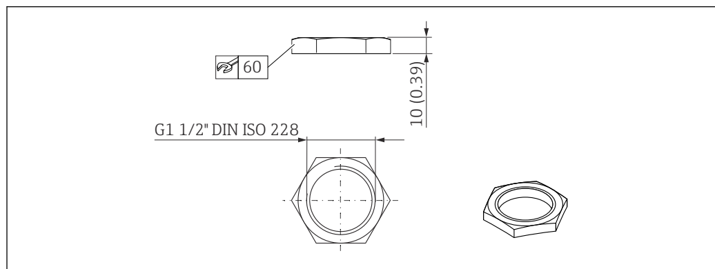
28 Abmessungen Befestigungsmutter. Maßeinheit mm (in)
