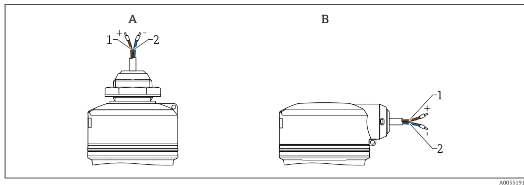
10 Kabelbelegung
