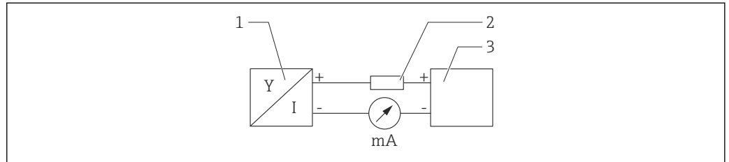
11 Blockschaltbild HART-Anschluss
