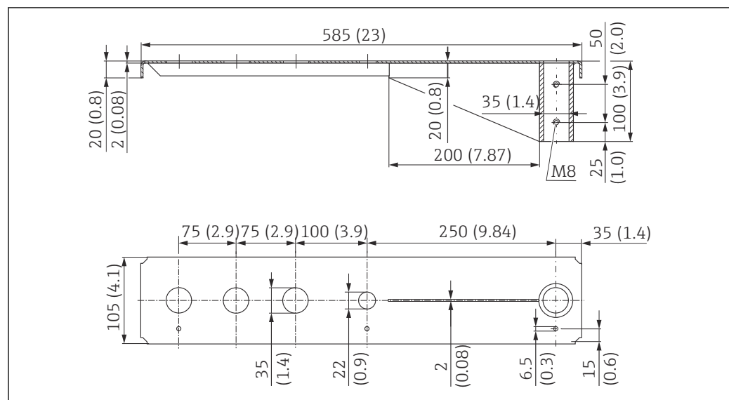
40 Abmessungen Ausleger 500 mm schwenkbar für Sensor Prozessanschluss Kabeleinführung. Maßeinheit mm (in)
