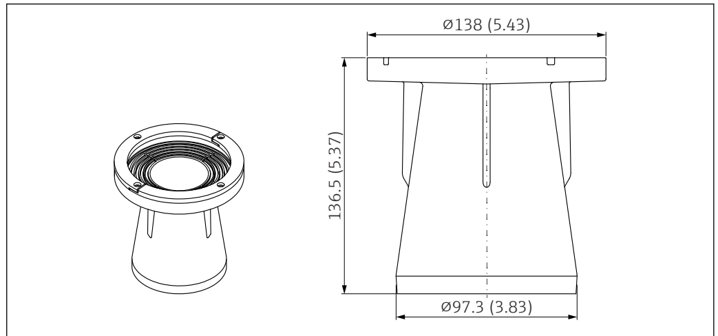
33 Abmessungen Überflutungsschutzhülse 80 mm (3 in). Maßeinheit mm (in)
