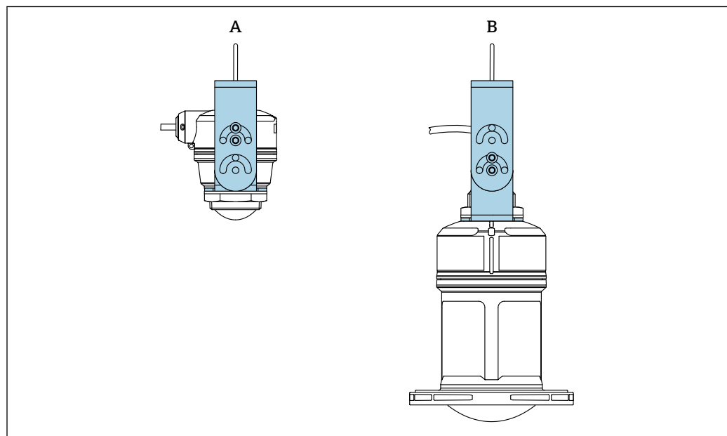
7 Einbau mit Seilmontage
