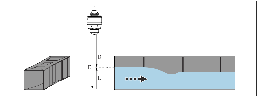
23 Beispiel: Khafagi-Venturi-Rinne
