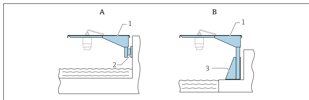
39 Montageart Sensor Prozessanschluss Kabeleinführung
