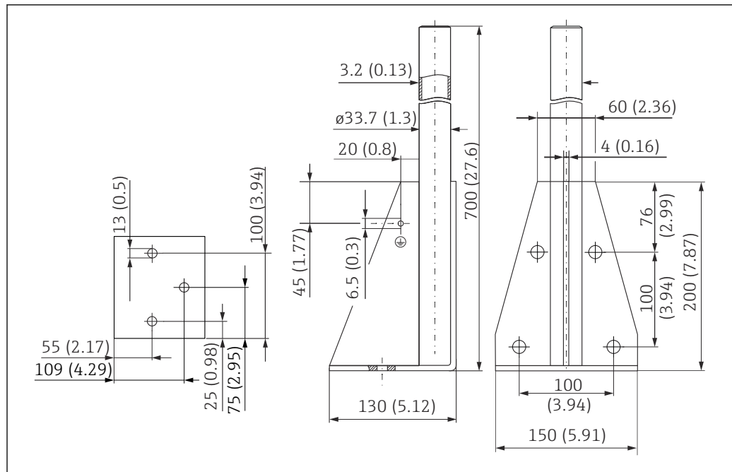
45 Abmessungen. Maßeinheit mm (in)
