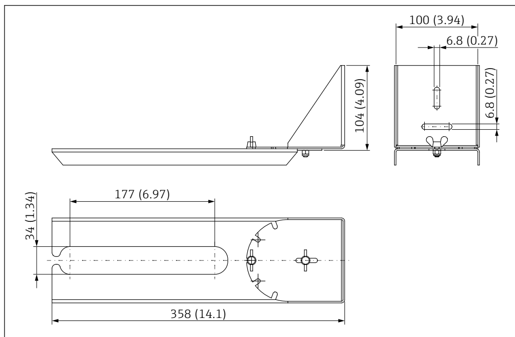
48 Abmessungen schwenkbare Montagehalterung. Maßeinheit mm (in)
