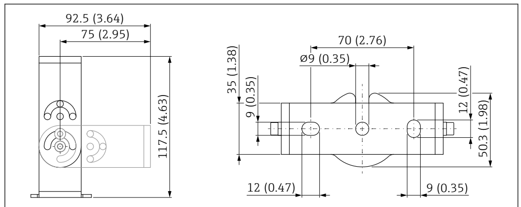
34 Abmessungen Montagebügel. Maßeinheit mm (in)
