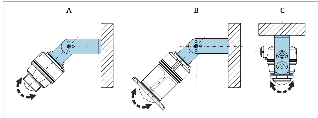
6 Einbau mit Montagebügel ausrichtbar
