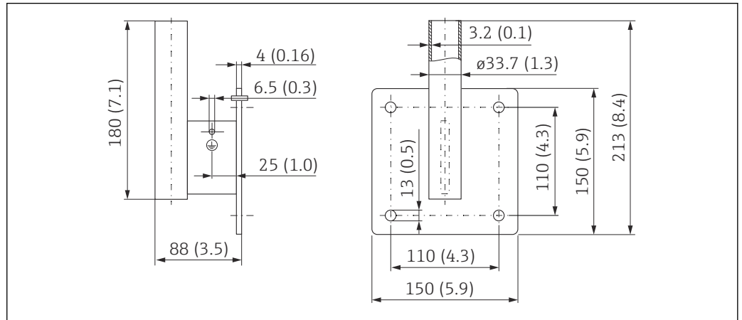
47 Abmessungen Wandhalter. Maßeinheit mm (in)
