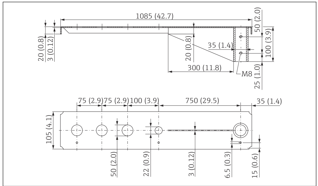
44 Abmessungen Ausleger 1 000 mm schwenkbar für Sensor Prozessanschluss Antennenende G 1½". Maßeinheit mm (in)
