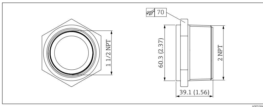
31 Abmessungen Adapter Uni
