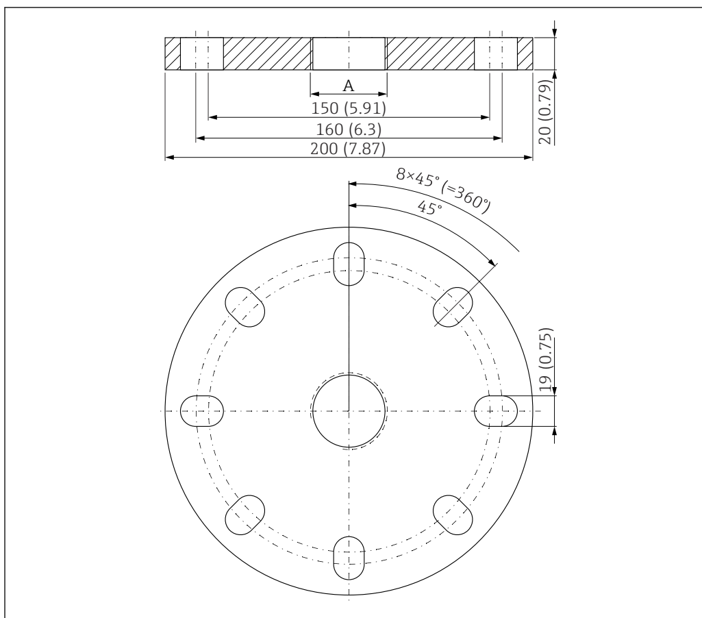
54 Abmessungen UNI Flansch 3"/DN80/80. Maßeinheit mm (in)
