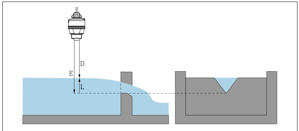
24 Beispiel: Dreieckswehr
