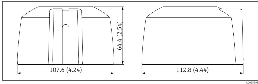
27 Abmessungen für Wetterschutzhaube mit Kabeleinführung seitlich. Maßeinheit mm (in)
