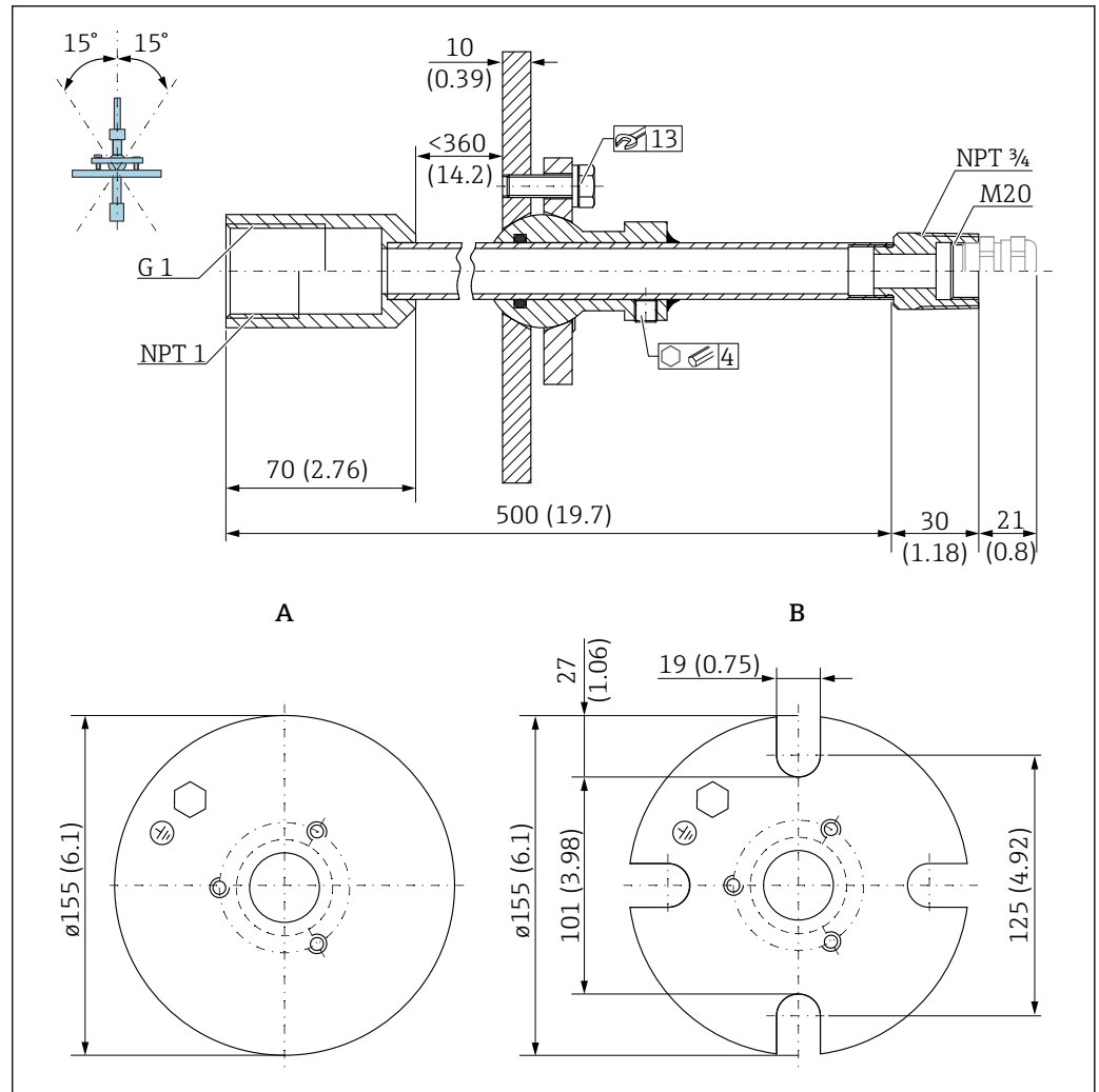
49 Abmessungen. Maßeinheit mm (in)
