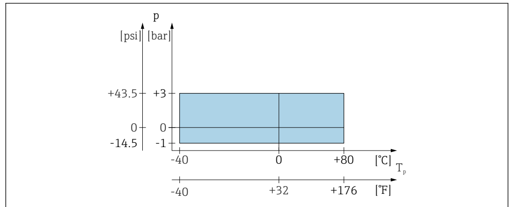
59 Zulässiger Bereich für Prozesstemperatur und Prozessdruck
