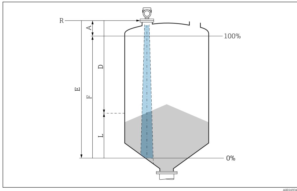
21 Konfigurationsparameter zur Füllstandmessung in Schüttgütern
