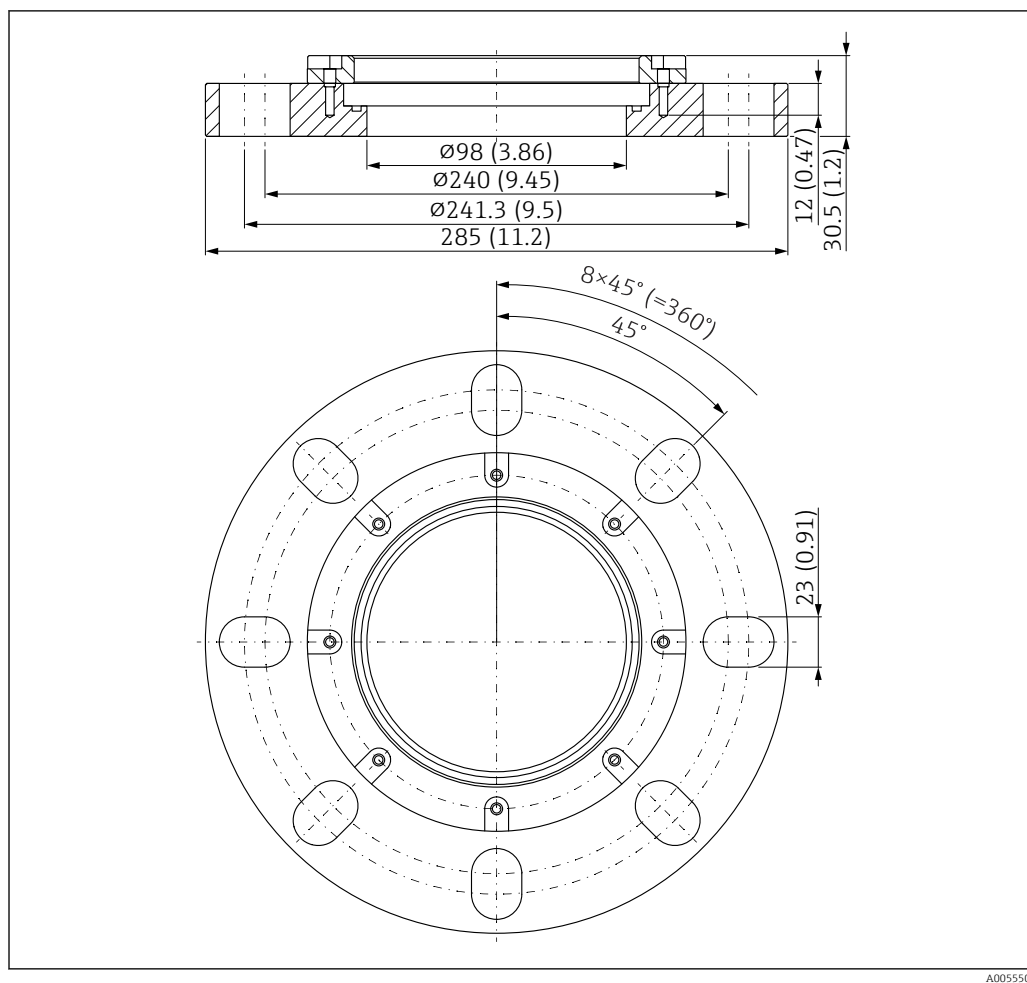
52 Abmessungen UNI-Überwurfflansch 6"/DN150/150. Maßeinheit mm (in)
