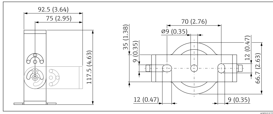
35 Abmessungen Montagebügel. Maßeinheit mm (in)
