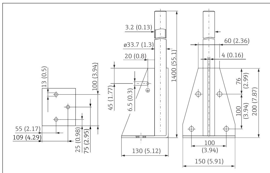
46 Abmessungen. Maßeinheit mm (in)
