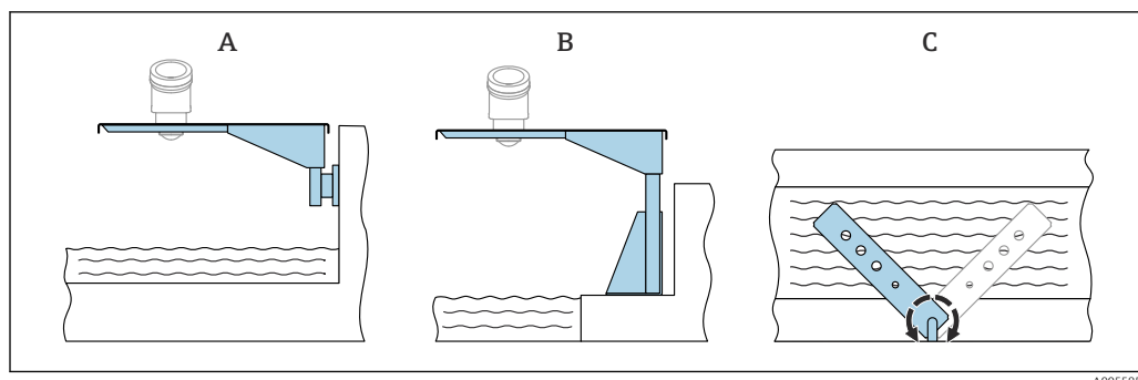
■ 16 Montage Ausleger schwenkbar
