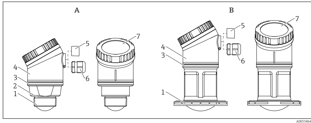
22 Geräteaufbau
