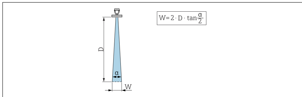
13 Zusammenhang zwischen Abstrahlwinkel \alpha , Distanz D und Kegelweite W
