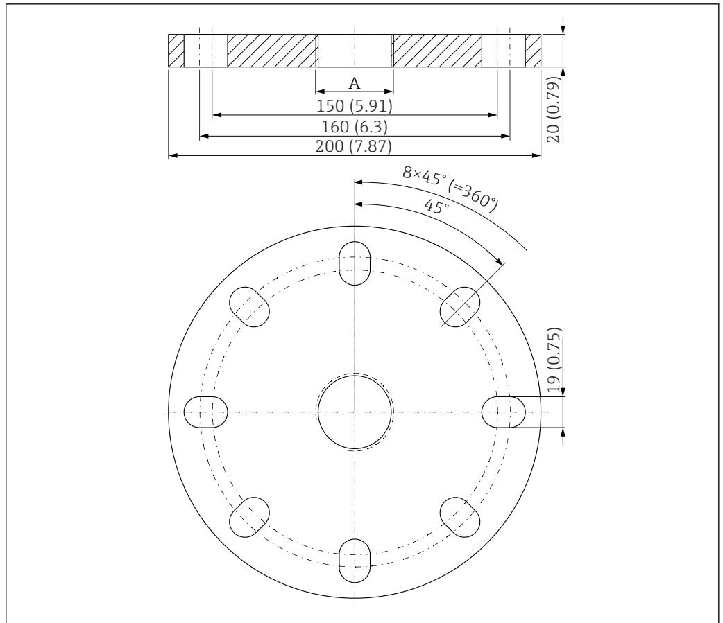
42 Abmessungen UNI Flansch 3\"/>
