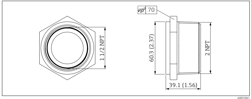
28 Abmessungen Adapter Uni
