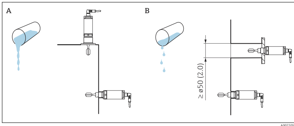
4 Einbaumöglichkeiten unter Berücksichtigung der Viskosität, Maßangabe mm (in)
