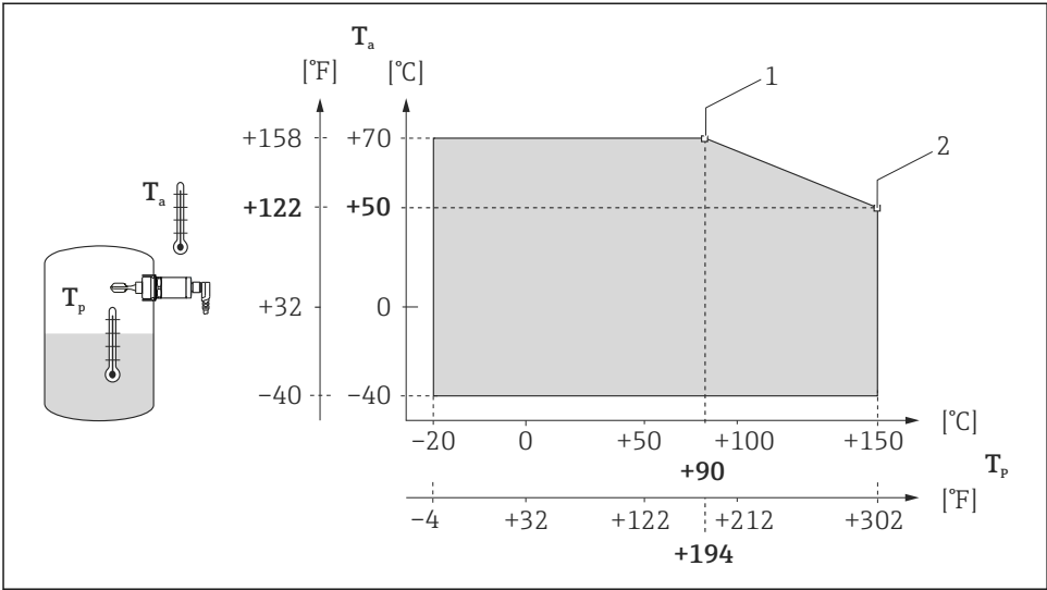
18 Derating-Kurve: 150 °C (302 °F)
