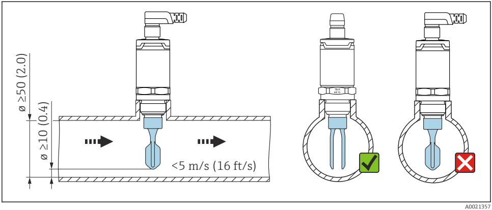
8 Stellung der Schwinggabel in Rohrleitungen. Maßeinheit mm (in)
