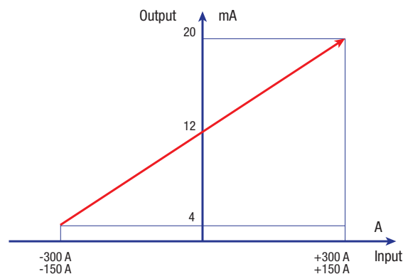
Input / Output
