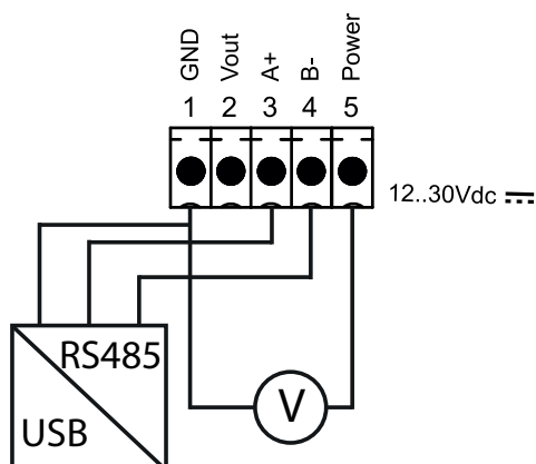
Anschlusschema BT7100
