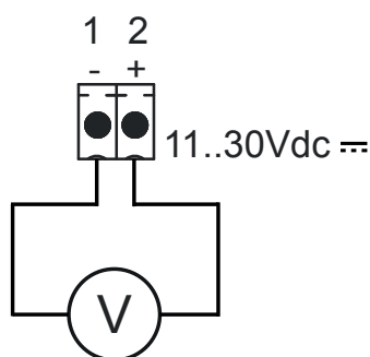
Anschlusschema BT7150
