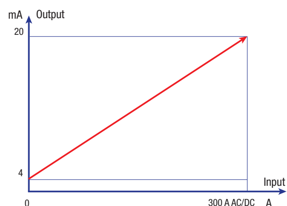
Input / Output
