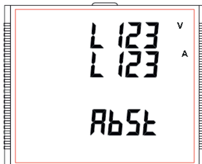
Alle drei Phasen (Spannung und Strom) fehlen
