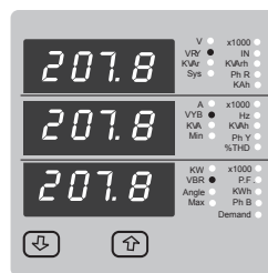
Anzeige 3: Leiter-zu- Leiter-Spannungen
