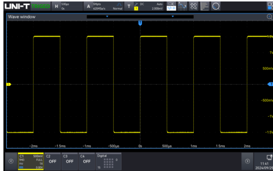
Nicht gemittelte Wellenform
