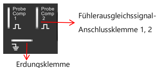
Anschlussklemme und Erdungsklemme für das Kompensationssignal des Tastkopfs
