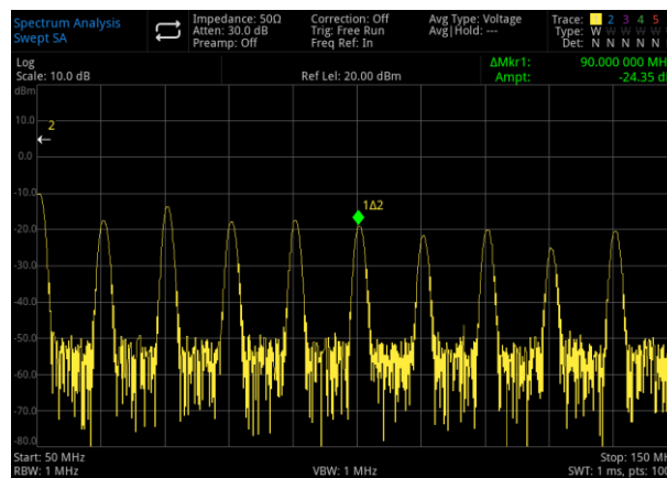
Abbildung 3-3 Differenzwertmarker des Referenzsignals außerhalb des Bildschirms
