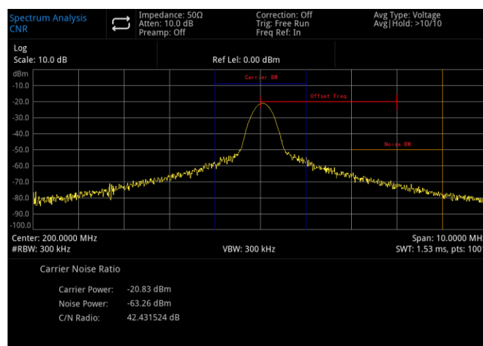
Abbildung 5-7 Messung des Träger-Rausch-Verhältnisses
