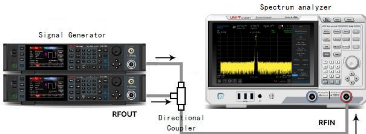
Abbildung 3-4: Geräteeinstellung für die Erfassung von zwei Kanalsignalen
