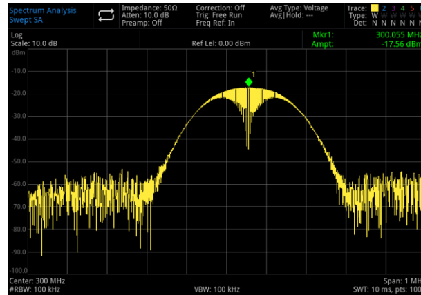
Abbildung 3-5 Zwei Signale mit gleicher Amplitude, die sich nicht unterscheiden
