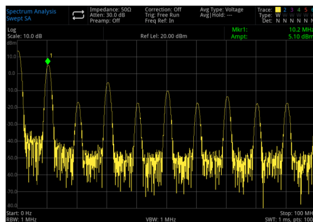
Abbildung 3-1 Frequenz und Amplitude lesen
