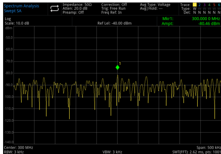
Abbildung 3-11 Ein Signal in der Nähe des Grundrauschens
