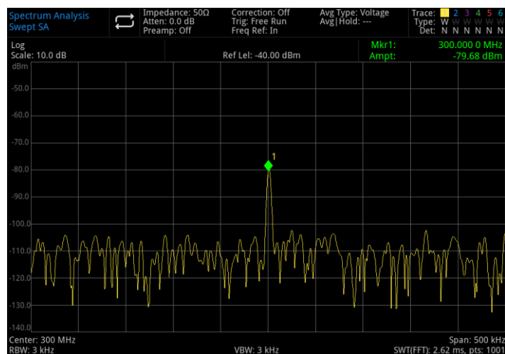
Abbildung 3-12 Messung kleiner Signale mit 0dB Dämpfung
