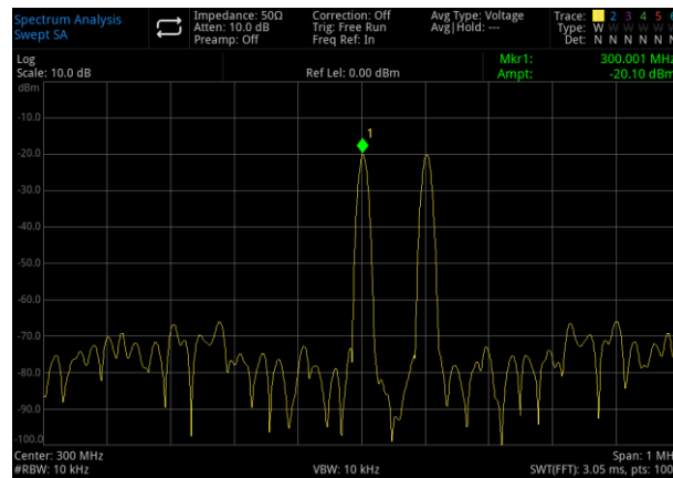
Abbildung 3-7 Zwei Signale mit gleicher Amplitude unterschieden (2)
