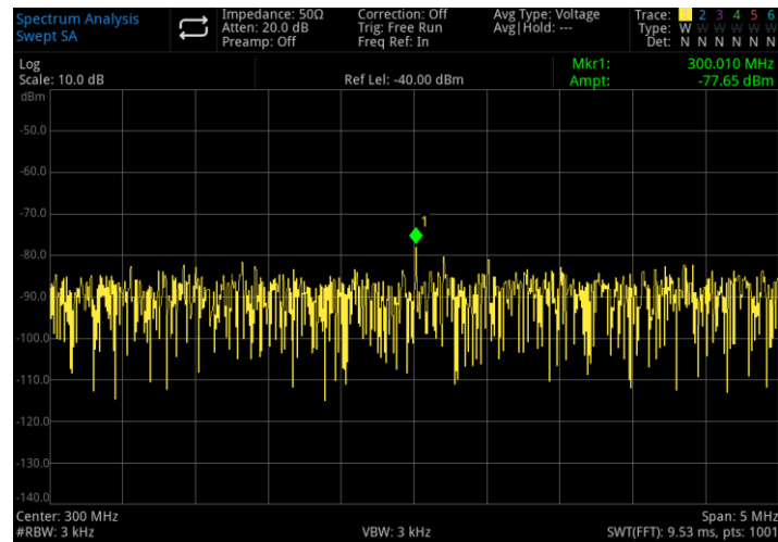
Abbildung 3-13 Bandbreite der Auflösung reduzieren
