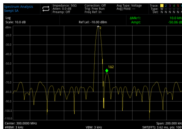
Abbildung 3-9: Unterscheiden Sie kleine Signale von großen Signalen
