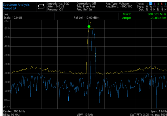
Abbildung 3-15 Maximales Halten und Aktualisieren zur Beobachtung der Signaldrift
