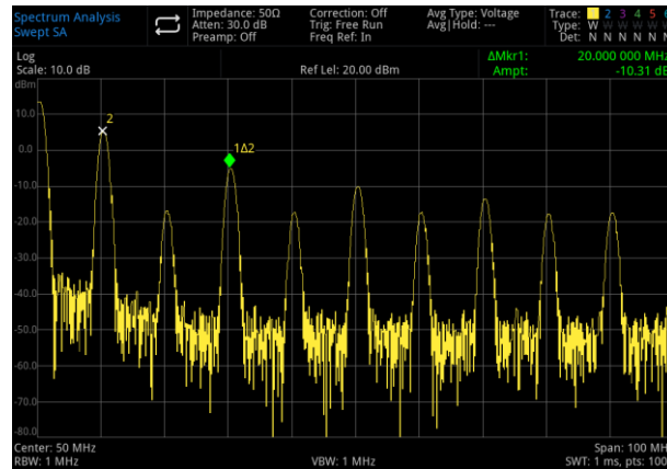
Abbildung 3-2 Marker-Modus Differenzwert \Delta auf dem gleichen Bildschirm zum Signalvergleich
