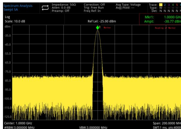
Abbildung 4-1 Ablesen des Markierungscursors
