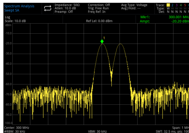
Abbildung 3-6 Zwei Signale mit gleicher Amplitude unterschieden (1)
