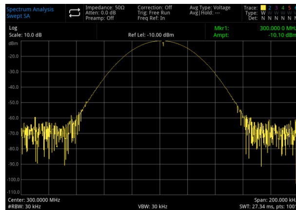
Abbildung 3-8: Kleines Signal nicht von großem Signal unterscheiden können
