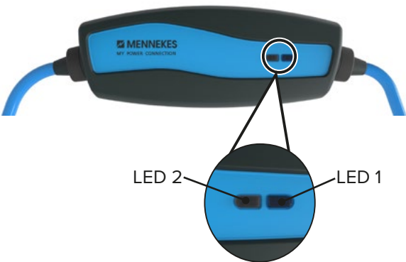
Imagen: Disposición de los LED en la parte superior del aparato
