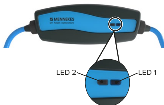
Figura: Disposição dos LED na parte superior do invólucro
