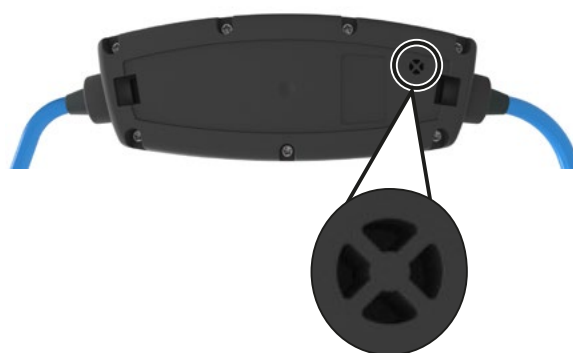
Figura: Orifício de purga na parte inferior do invólucro
