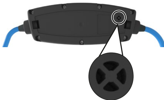
Bild: Öppning för avluftning av höljets undersida
