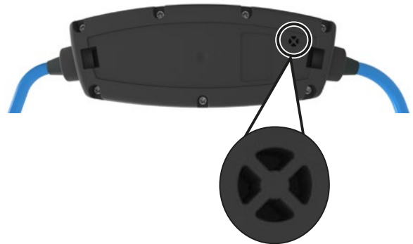
Kuva: Tuuletukseen tarkoitettu aukko kotelon pohjassa
