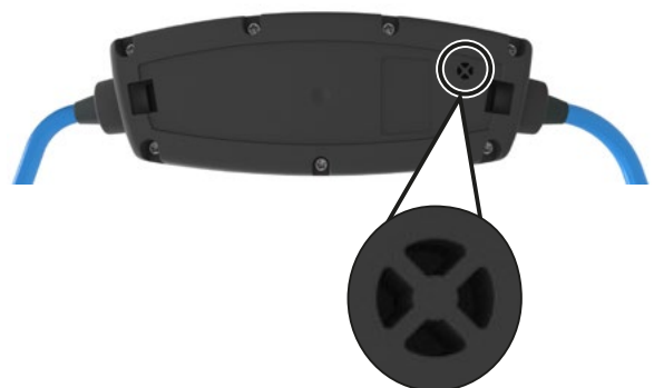
Εικόνα: Στόμιο για τον εξαερισμό στην κάτω πλευρά του περιβλήματος
