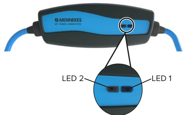
Figura: colocación de los LEDs en la parte superior de la carcasa
