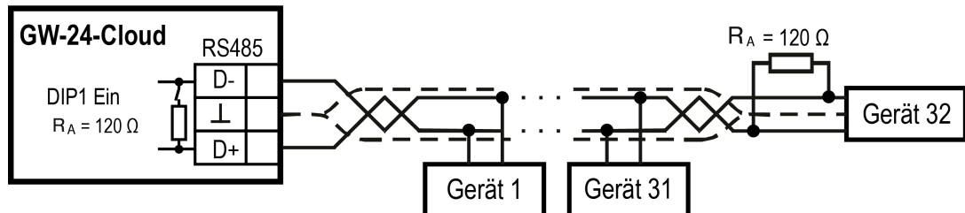
Abb. 7.2 RS485-Schlittstelle
