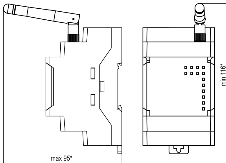
Abb. 6.2 Abmessungen des Geräts mit angeschlossener Antenne
