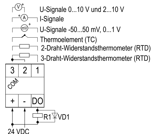
Abb. 6 Anschlussdiagramm
