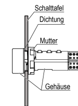
Abb. 1 Montage
