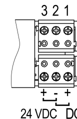
Abb. 5 Klemmenbelegung
