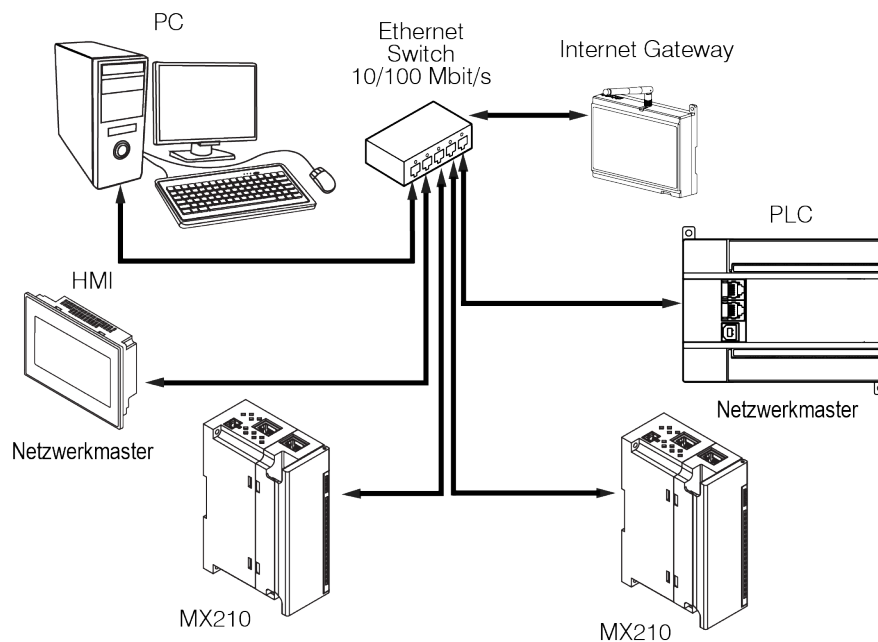
Abb. 5.7 Stern-Topologie
