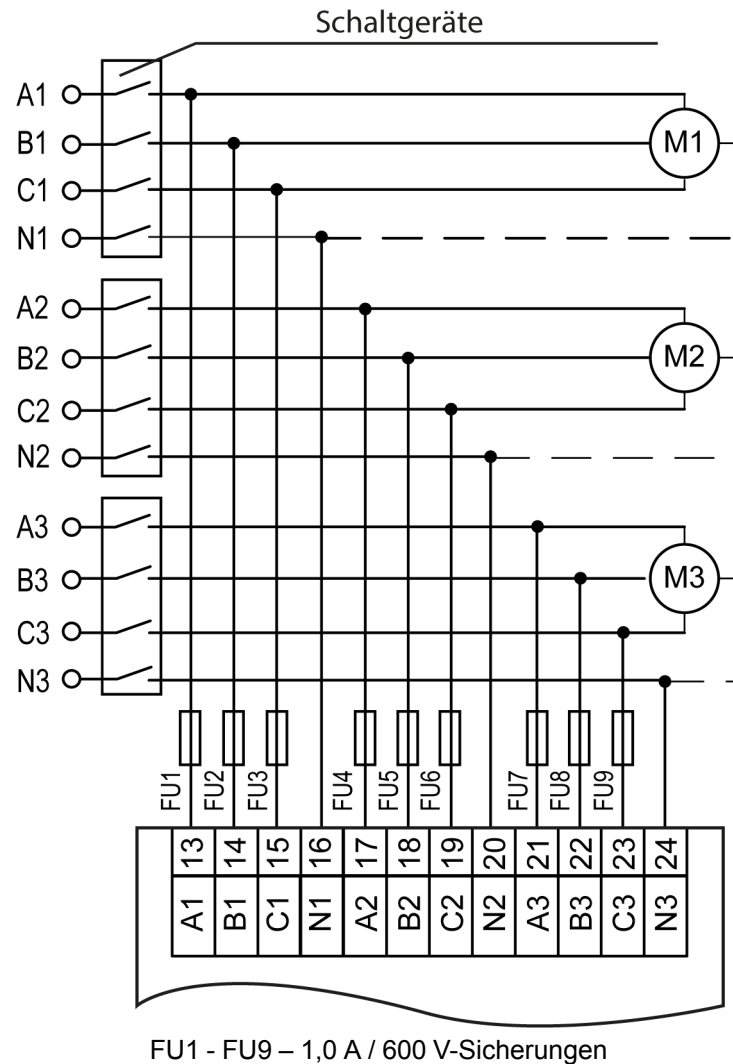
Abb. 5.6 Anschluss von dreiphasigen Stromkreisen
