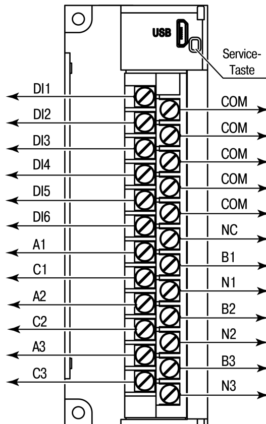
Abb. 5.3 Frontansicht (offene Abdeckung)
