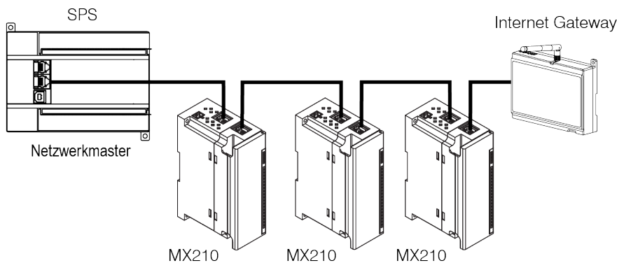
Abb. 5.8 Chain-Topologie
