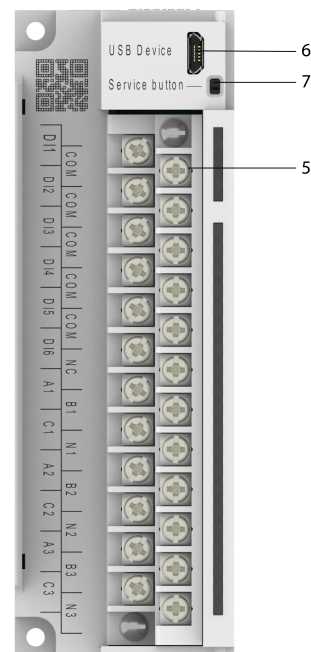
Abb. 2.2 Frontansicht (Ausene Abdeckung)
