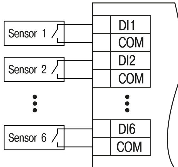
Abb. 5.4 Anschluss von Schaltkontakten
