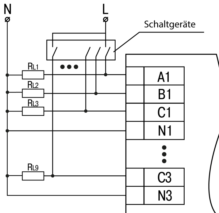
Abb. 5.5 Anschluss von einphasigen Stromkreisen
