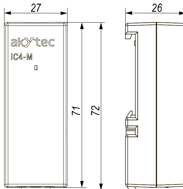
Abb. 1 Abmessungen
