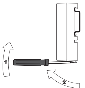
Abb. 4 Demontage
