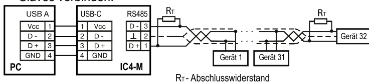
Abb. 5 Anschlussplan
