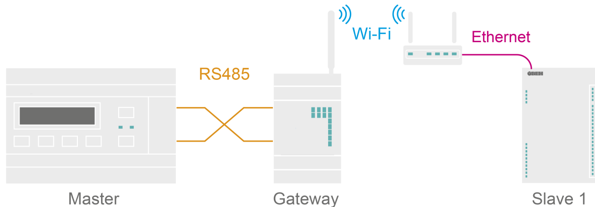
Abb. A.1 Anschlussdiagramm
