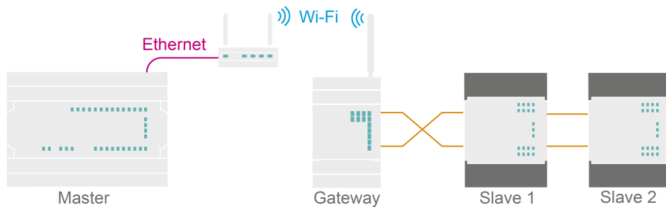
Abb. 8.12 Verwendung des Gateways mit Slave-Geräten in der RS485-Schnittstelle
