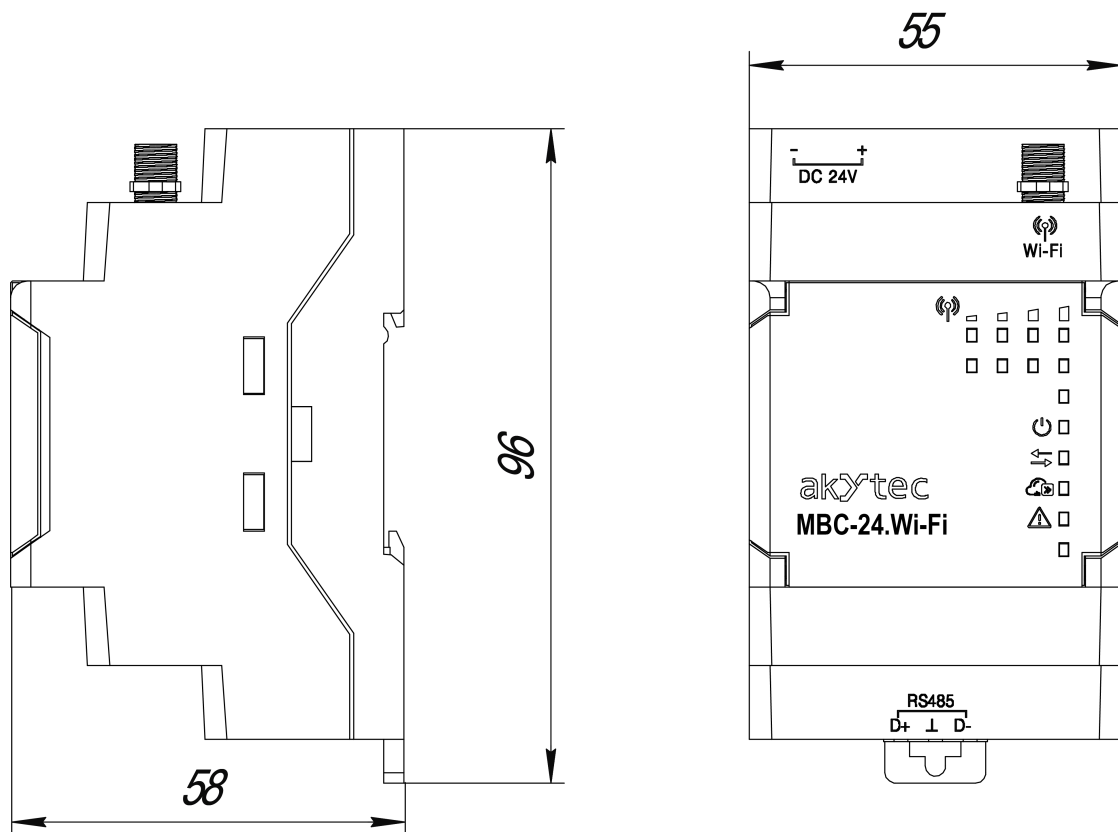
Abb. 5.1 Abmessungen
