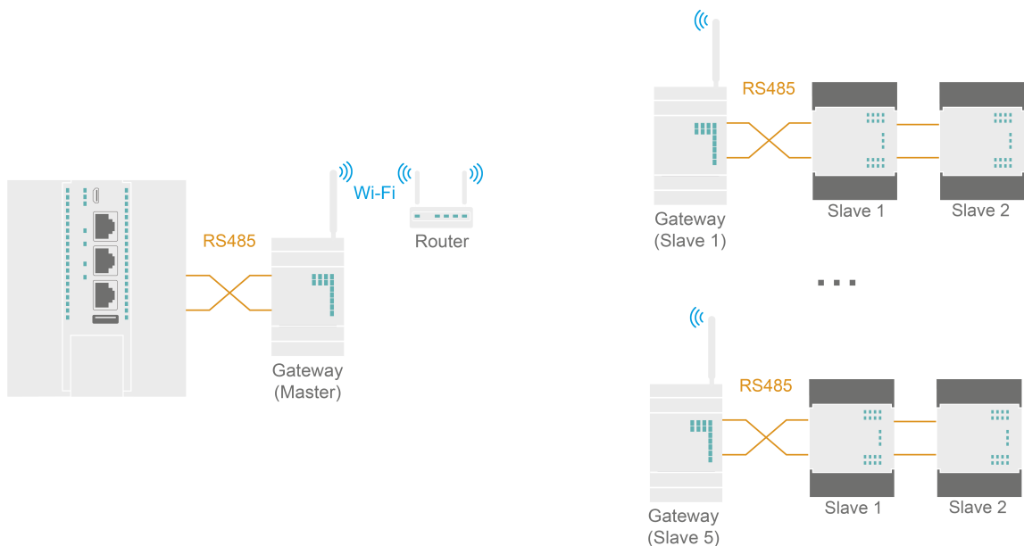
Abb. 8.13 Sterntopologie unter Verwendung eines externen Routers
