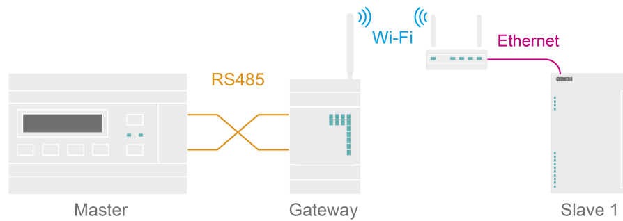
Abb. 8.11 Verwendung des Gateways mit Master in der RS485-Schnittstelle
