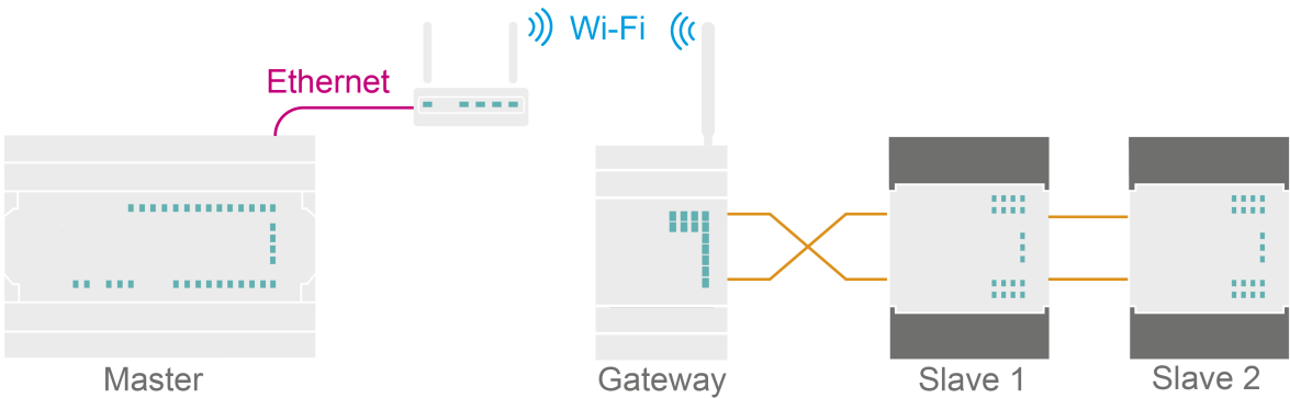
Abb. A.2 Anschlussdiagramm
