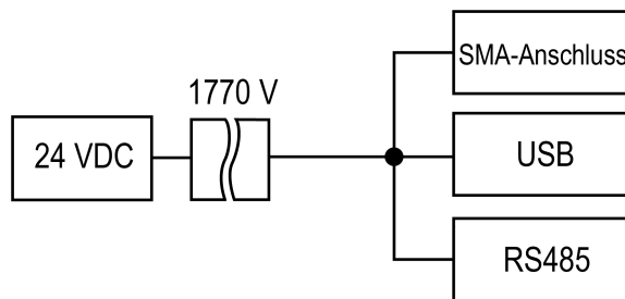
Abb. 3.1 Galvanische Trennung
