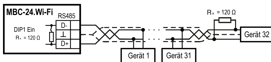
Abb. 6.1 RS485–Netzwerk
