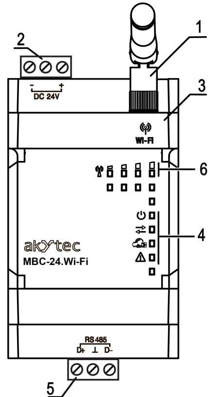
Abb. 7.1 Frontansicht
