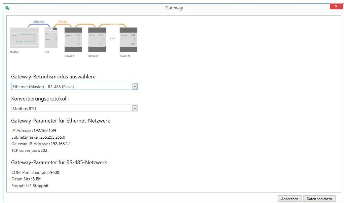
Abb. 8.14 Gateway-Konfigurationen im Modus Master in Wi-Fi - Slave in RS485
