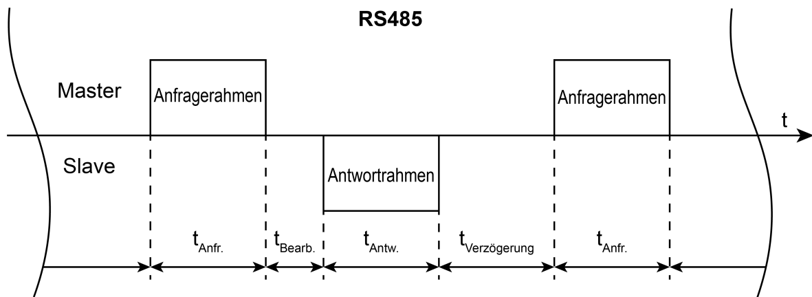
Abb. 8.10 Betriebsdiagramm des Parameter "Verzögerung zwischen den Paketen"
