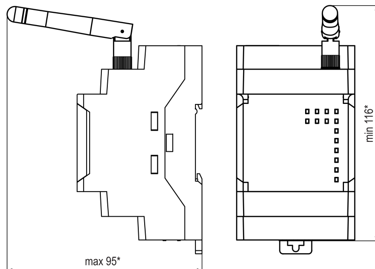
Abb. 5.2 Abmessungen des Geräts mit angeschlossener Antenne
