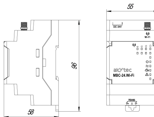
Abb. 1 Abmessungen
