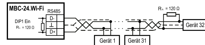
Abb. 2 Anschluss
