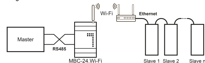
Abb. 3 Verwendung des Gateways mit Master in der RS485-Schnittstelle
