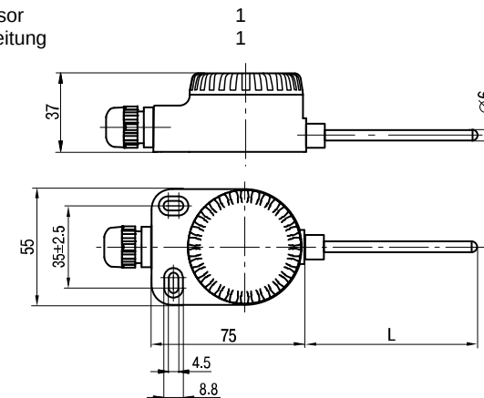
Abb. 2 Abmessungen
