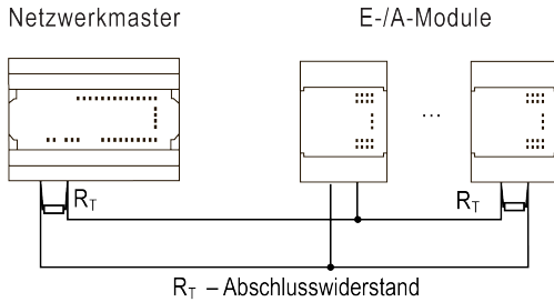
Abb. 13 PR103 als Master
