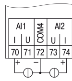
Abb. 6 Verdrahtung der Stromsensoren
