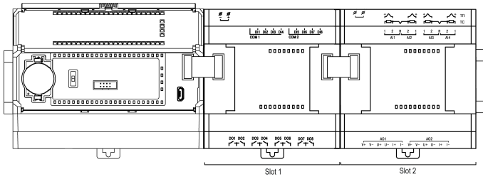
Abb. 11 Verdrahtung der Erweiterungsmodule
