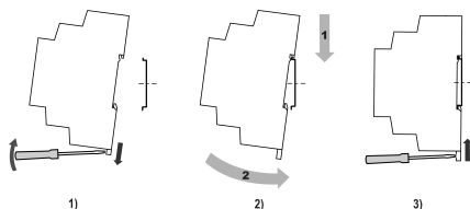
Abb. 2 Montage
