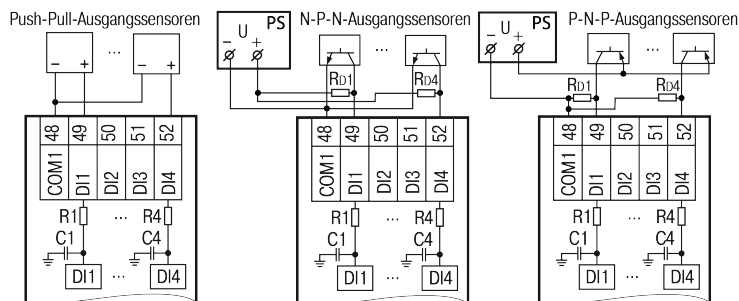
Abb. 3 Verdrahtung der Digitaleingänge
