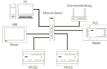
Abb. 14 Stern-Topologie
