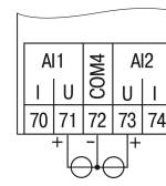
Abb. 7 Verdrahtung der Spannungssensoren
