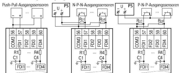
Abb. 8 Verdrahtung der schnellen Digitaleingänge
