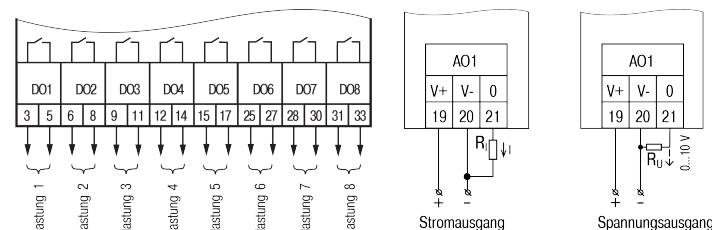
Abb. 9 Verdrahtung der Relaisausgänge
