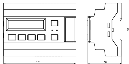
Abb. 1 Abmessungen
