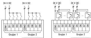
Abb. 6 Verdrahtung der Digitaleingänge (24 V AC)
