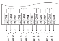
Abb. 8 Relaisausgänge
