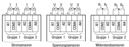
Abb. 7 Verdrahtung der Analogeingänge
