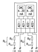
Abb. 9 Stromausgänge
