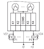
Abb. 11 Transistor-Optokopplerausgang
