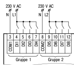
Abb. 5 Verdrahtung der Digitaleingänge (230 V AC)
