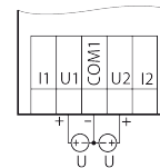
Abb. 7 Verdrahtung der Spannungssensoren
