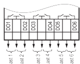
Abb. 10 Relais-Ausgänge
