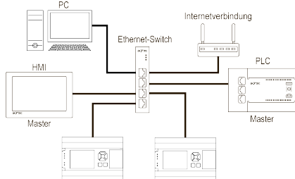
Abb. 15 Stern-Topologie
