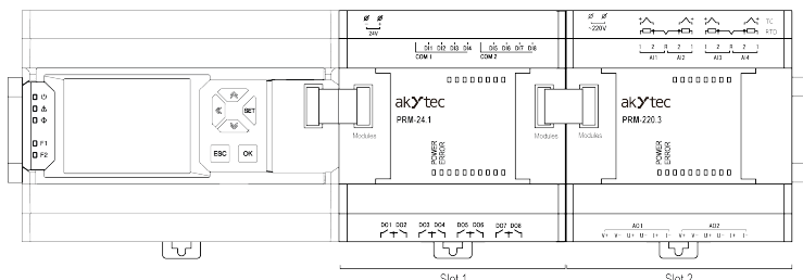
Abb. 16 Verdrahtung der Erweiterungsmodule
