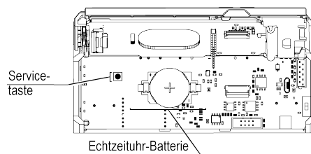
Abb. 18 Elemente unter der Frontplatte
