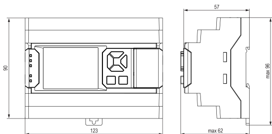
Abb. 1 Abmessungen
