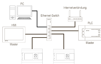
Abb. 14 Stern-Topologie
