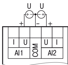
Abb. 5 Spannungssensoren
