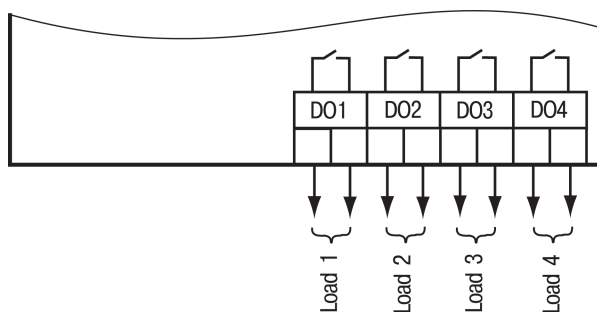
Abb. 9 Relaisausgänge
