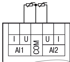
Abb. 3 RTD-Sensoren
