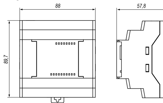
Abb. 11 Abmessungen
