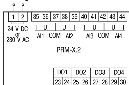
Abb. 2 Klemmenanordnung
