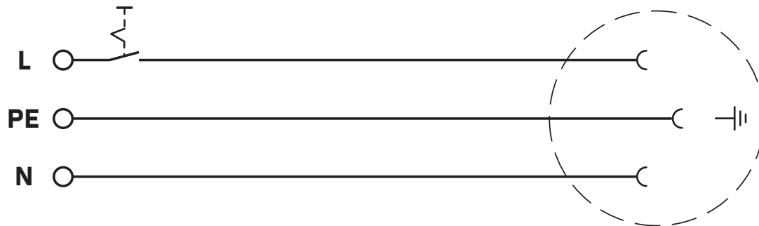
Schaltplan
