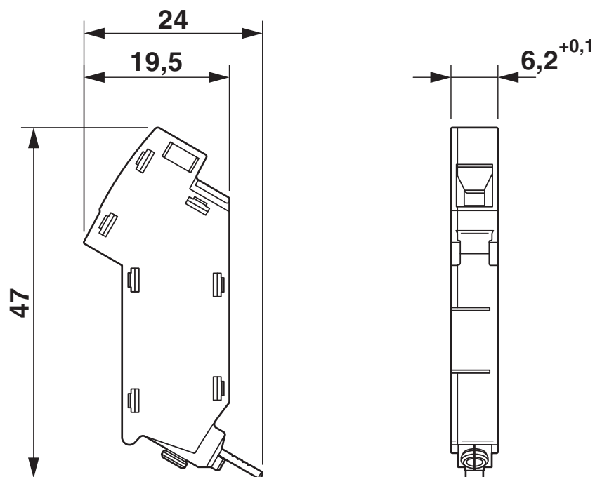
Maßzeichnung
