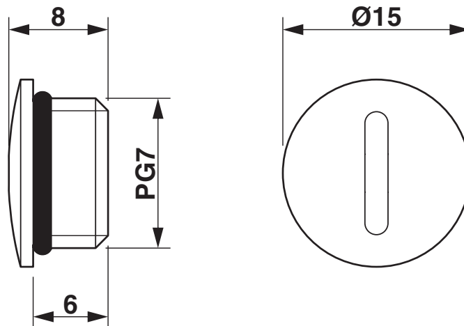
Maßzeichnung
