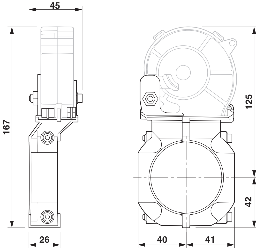
Maßzeichnung
