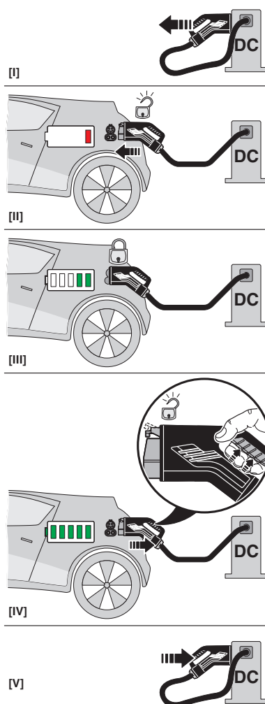
Schemazeichnung
