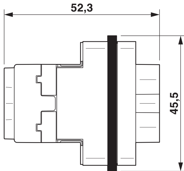
Maßzeichnung
